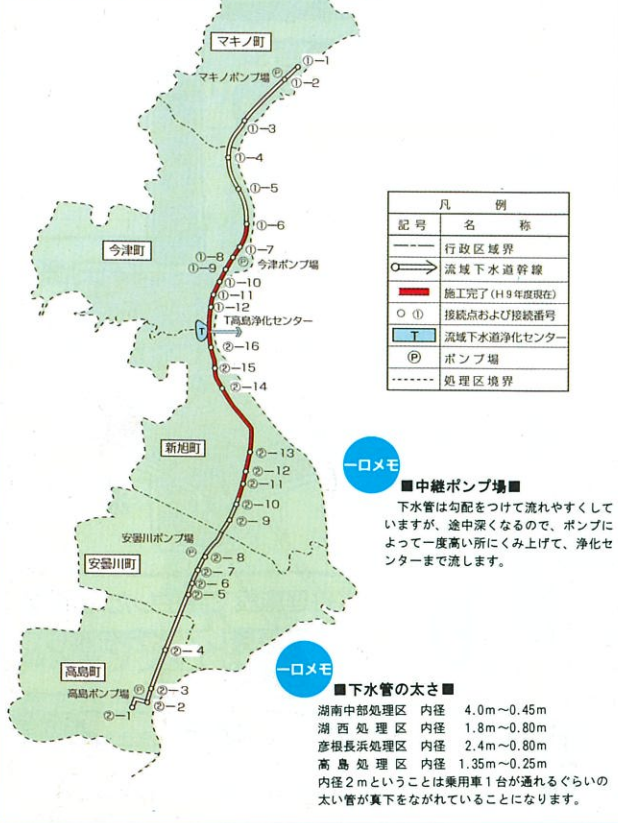
高島処理区幹線管渠およびポンプ場図
