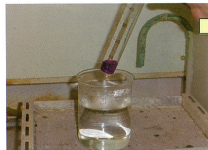
過マンガン酸カリウム溶液、硫酸、試料を入れ、沸とう水に入れる前の状態
