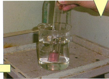
過マンガン酸カリウム溶液、硫酸、試料を入れ、沸とう水に入れた後の状態
